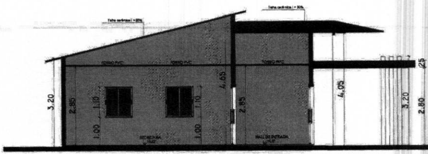
7 CORTE LONGITUDINAL BB
