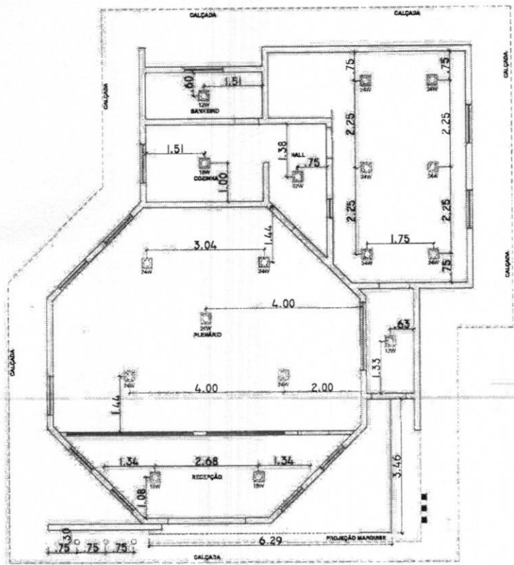
9 PONTOS DE LUZ 150
