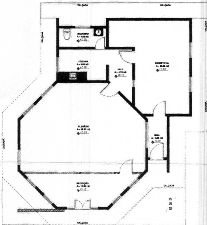
2 PLANTA DE DEMOLIÇÃO 1:50
