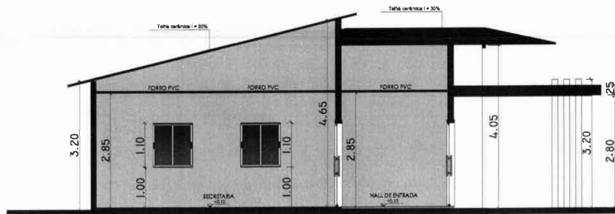
7 CORTE LONGITUDINAL BB 1/100
