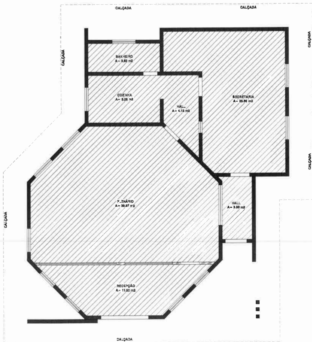
8 PLANTA DE FORRO 1:50
