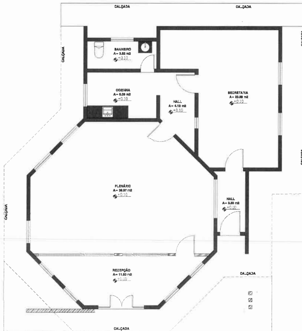
2 PLANTA DE DEMOLIÇÃO 1:50
