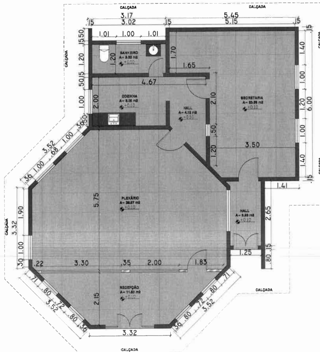
1 PLANTA BAIXA EXISTENTE 1:50
