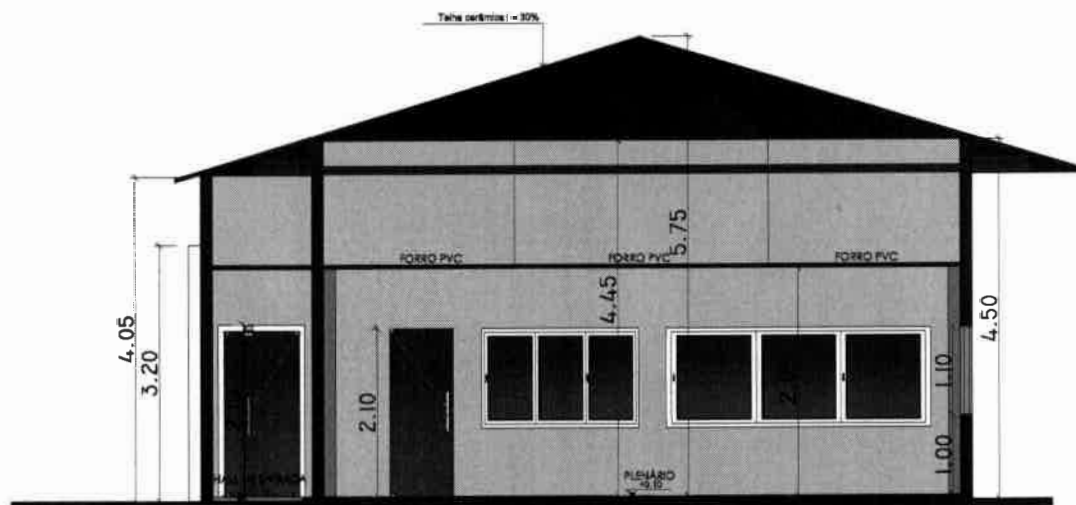
7 CORTE TRANSVERSAL AA 1/100
