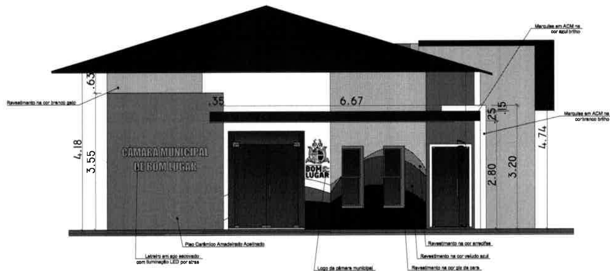
6 FACHADA 1:50
